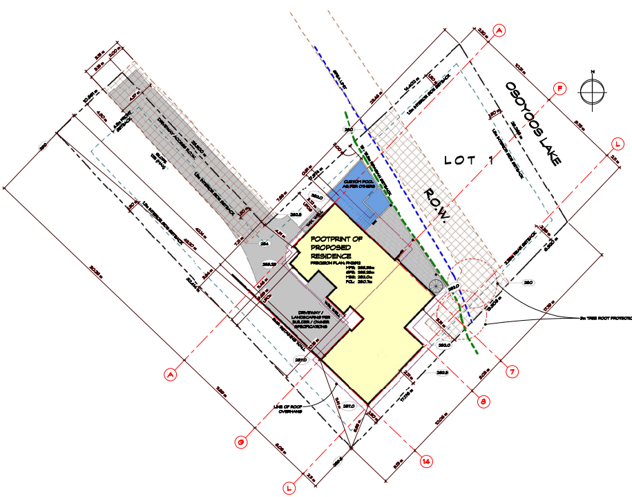
SITE PLAN 1:50
